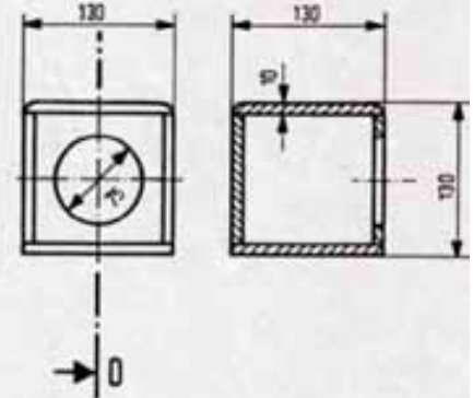
SCHNITT C-D
